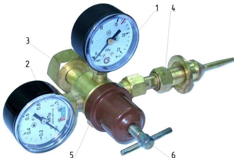
Рис.1 Редуктор БГО-5
